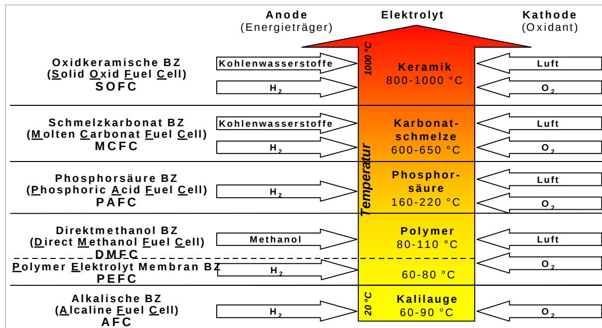
Abb. 2: Brennstoffzellentypen
