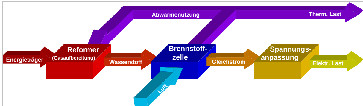
Abb. 3: Basiskomponenten eines Brennstoffzellensystems für kohlenstoffhaltige Energieträger
