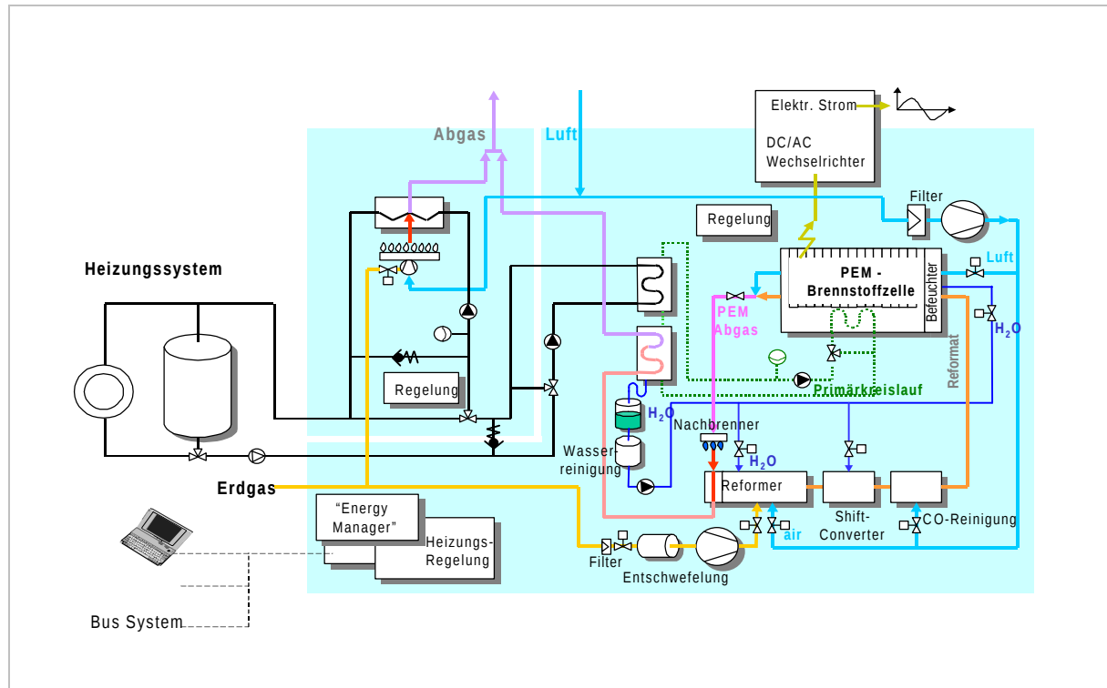
Abb. 1: Prozessflussdiagramm des Vaillant Brennstoffzellen-Heizgerätes
