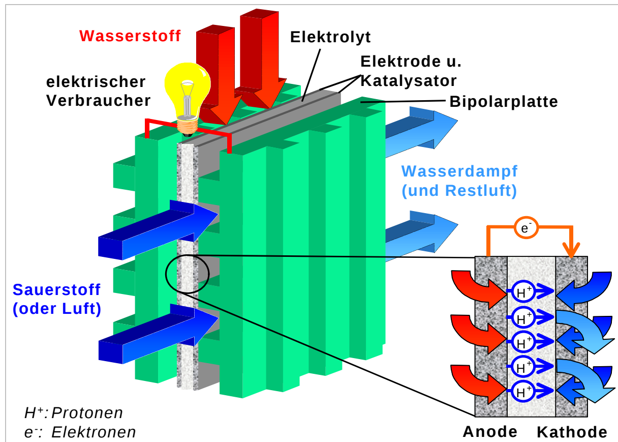
Abb. 1: Aufbau einer Brennstoffzelle
