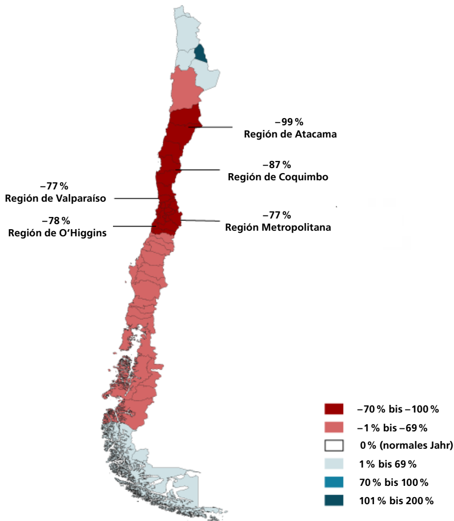
Abbildung 1 Karte der kumulierten Niederschlagsverluste/-überschüsse von August 2019*
